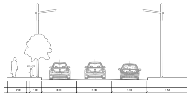
Profil stradal propus Str. 20 Decembrie 1989 conform SF "Reorganizarea circulației rutiere pe inelul I..." aprobat prin HCL 427/16.10.2015
