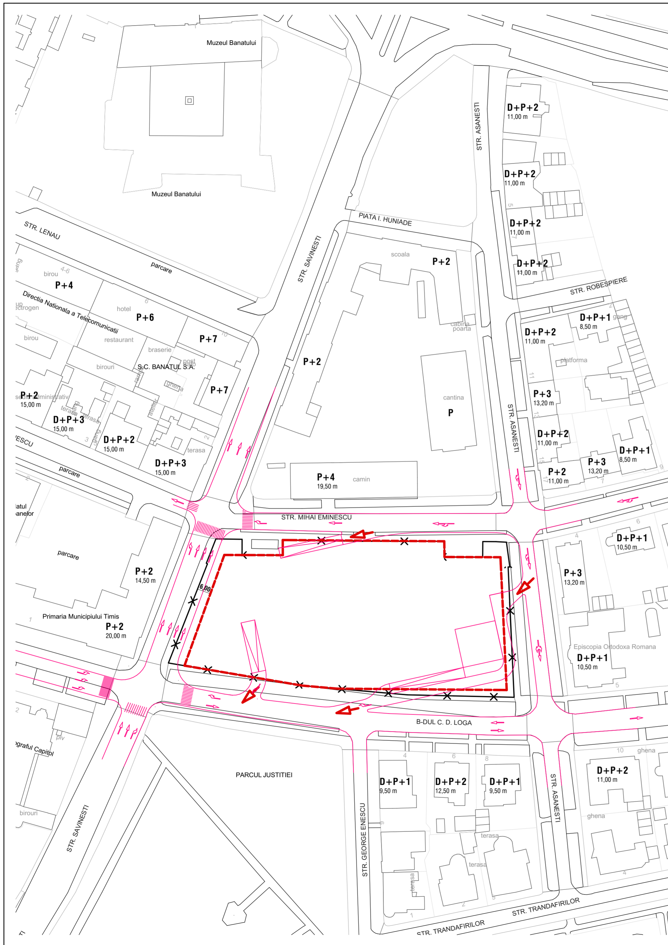
Circulații rutiere. Propunere. Scara 1:1000
