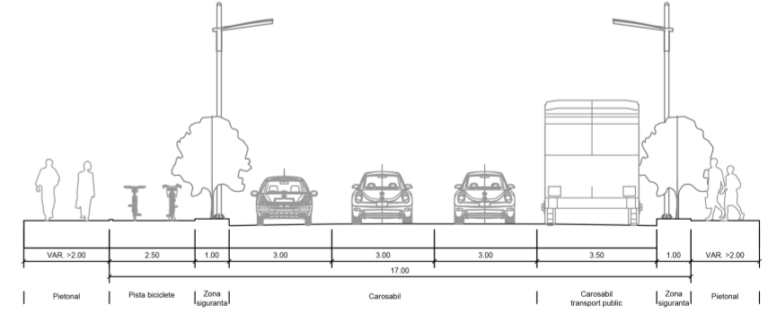
Profil stradal propus Str. 20 Decembrie 1989 conform SF "Reorganizarea circulației rutiere pe inelul I..." aprobat prin HCL 427/16.10.2015
